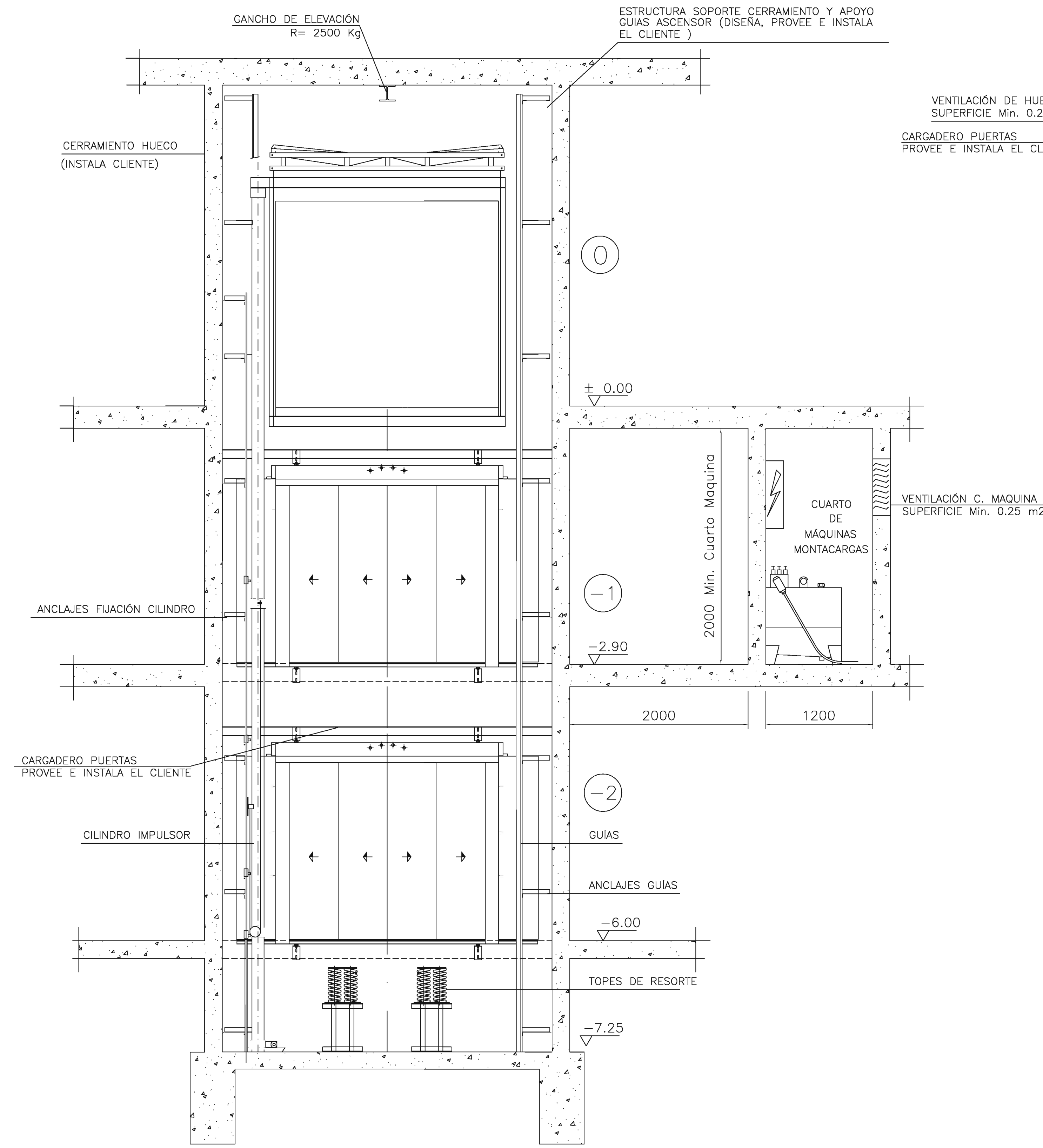
ALZADO SECCION A-A
