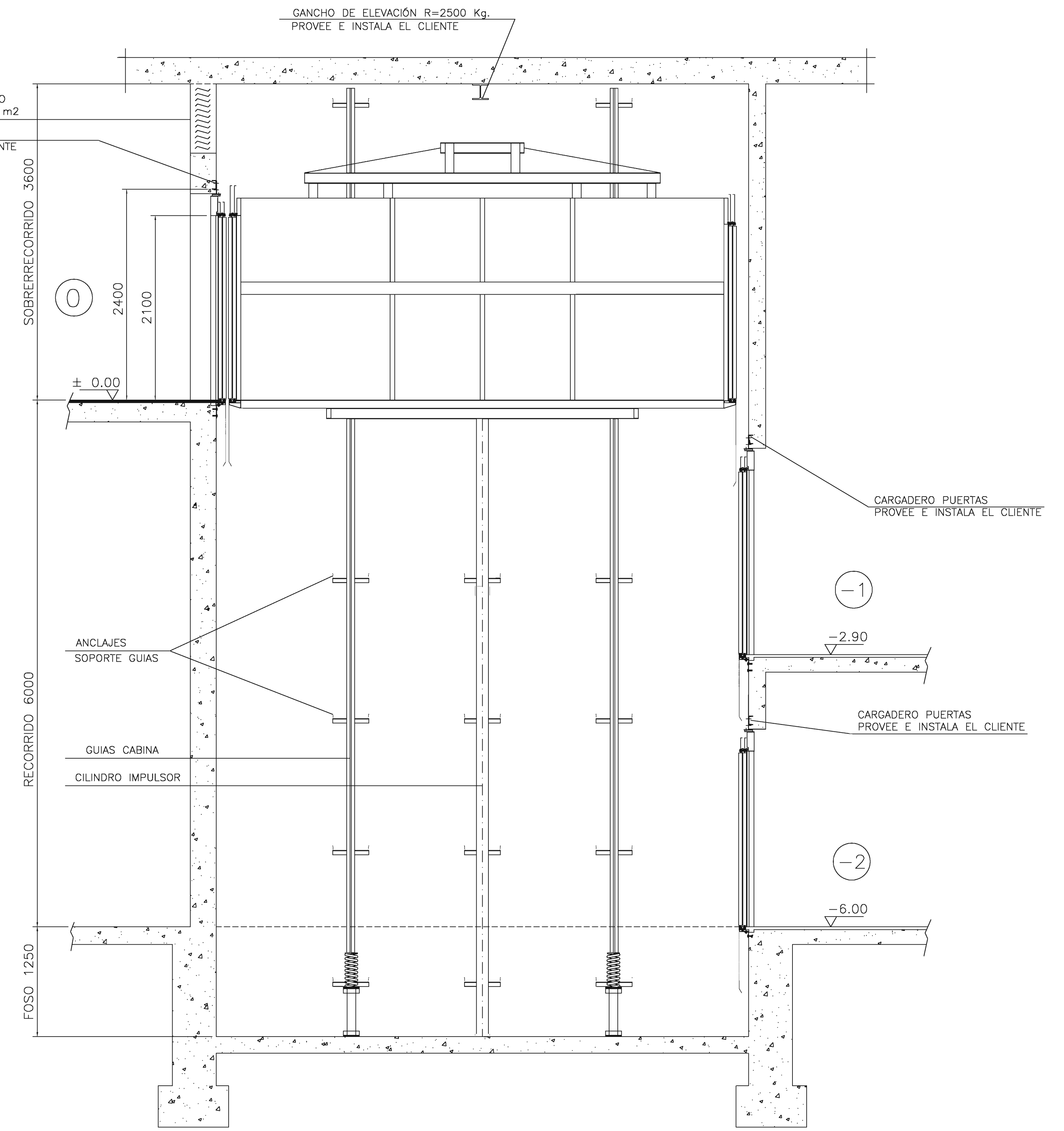
ALZADO SECCION B-B
